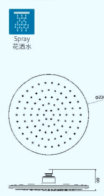
B26111 9" Rain shower 9寸圆形顶喷
