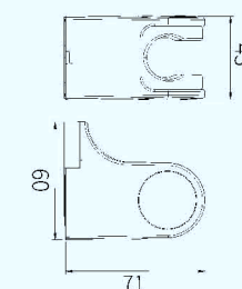
F42701 Adjustable wall bracket 可调式墙座
