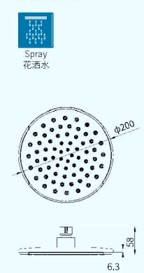
B27211 8" Rain shower 8寸圆形顶喷
