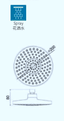
B25211 8" Rain shower 8寸圆形顶喷
