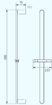
E36231 Shower set 方形升降杆 30*10mm
