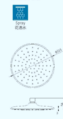
B27811 8" Rain shower 8寸圆形顶喷
